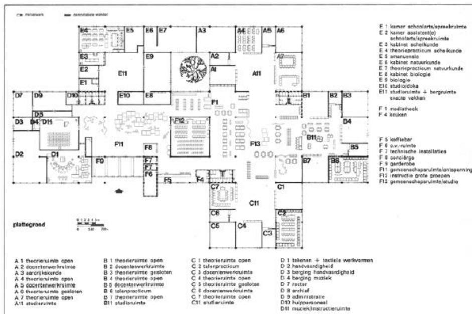
Plattegrond van het 'schoollandschap', 1973 (BOUW, nr. 19, 12-05-1973)
